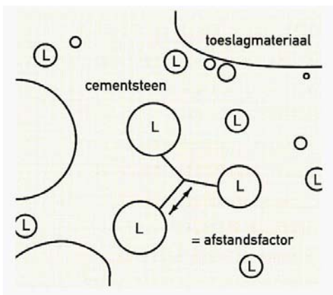
Figuur 4 Schematische weergave van de verdeling van luchtbellens (L) in beton en de afstandsfactor
