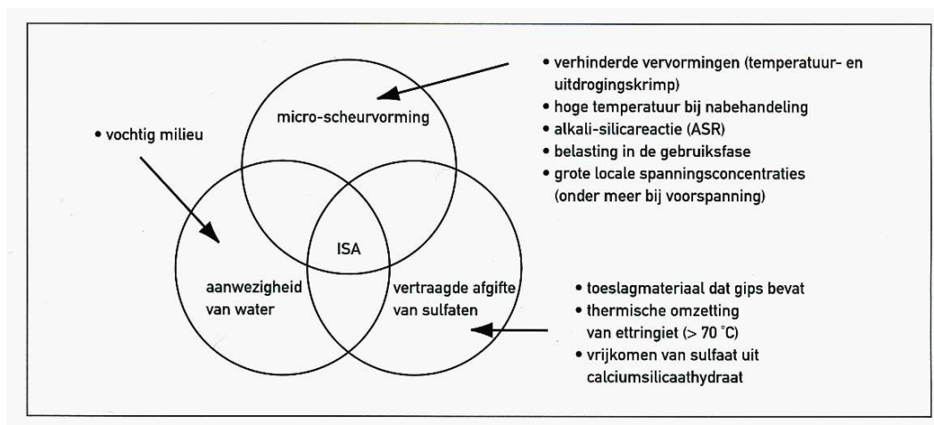
Figuur 3 Conditie waaronder interne sulfaataantasting (ISA) kan optreden
