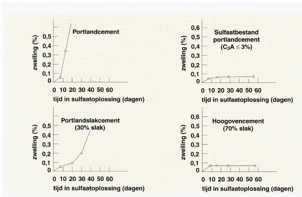
Figuur 4 Effect van gehalte aan hoogovenslak op de gevoeligheid van een cement voor sulfaataantasting
