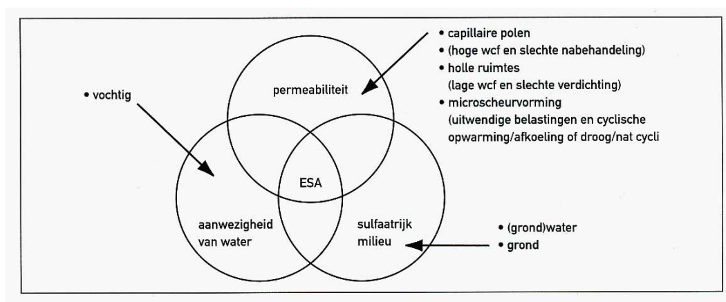
Figuur 1 Condities waaronder externe sulfaataantasting (ESA) kan optreden
